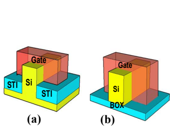
Fig. 1 (a) Bulk MG-FET (b) SOI MG-FET
